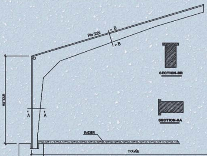
PORTIQUE NORMAL
