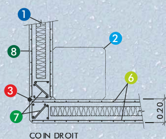
COIN DROIT
