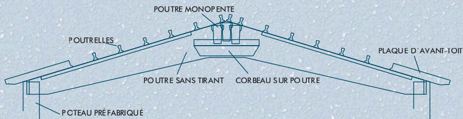
POUTRE MONOPENTE
